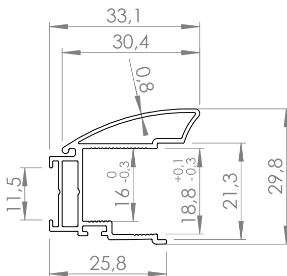
Aufrechtes Profil/Griffschiene SIGMA 8010 Rahmentyp C
