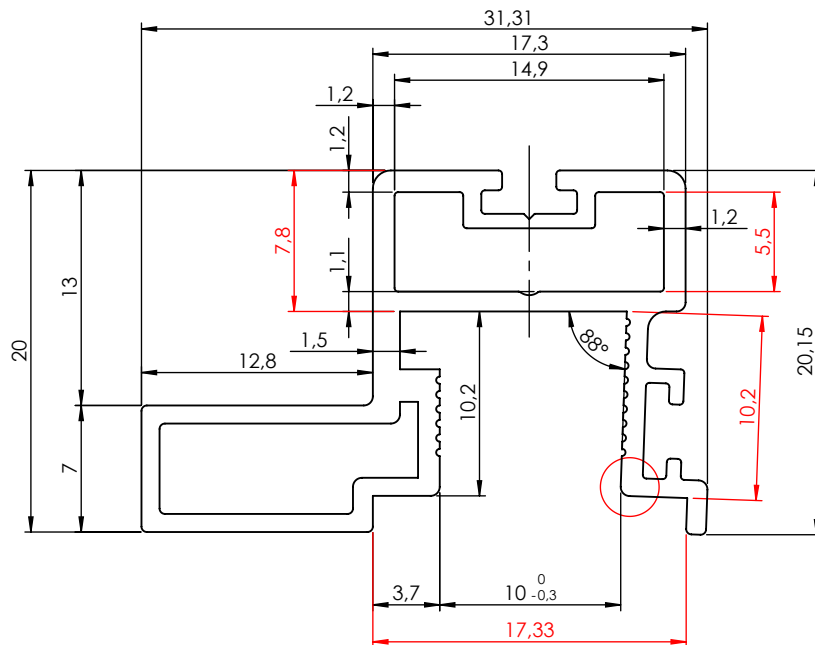
Aufrechtes Profil/Griffschiene BS Komfort Rahmentyp B/GALA 84200
