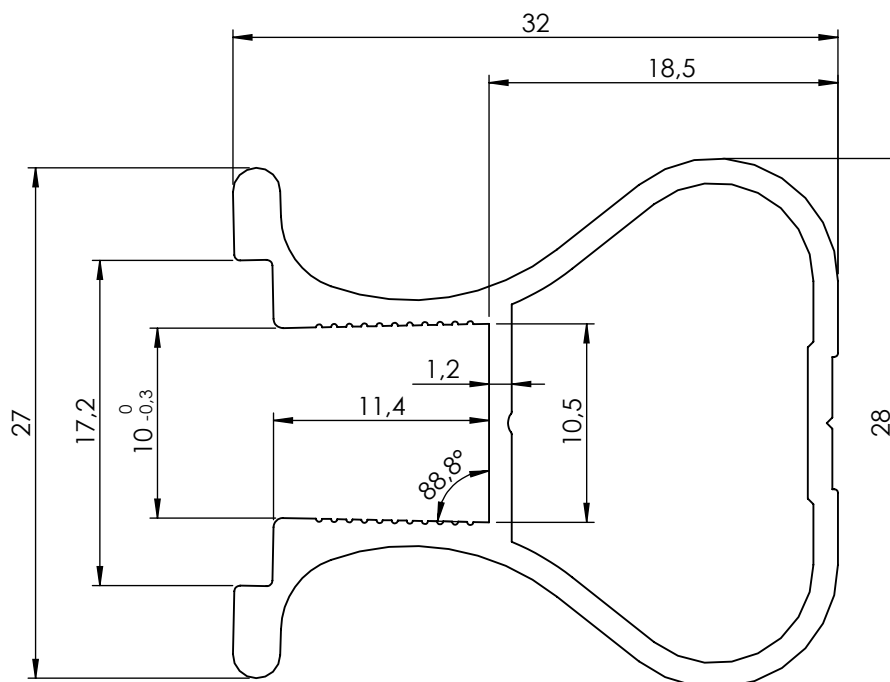
Aufrechtes Profil/Griffschiene LIMA 84700 Rahmentyp E
