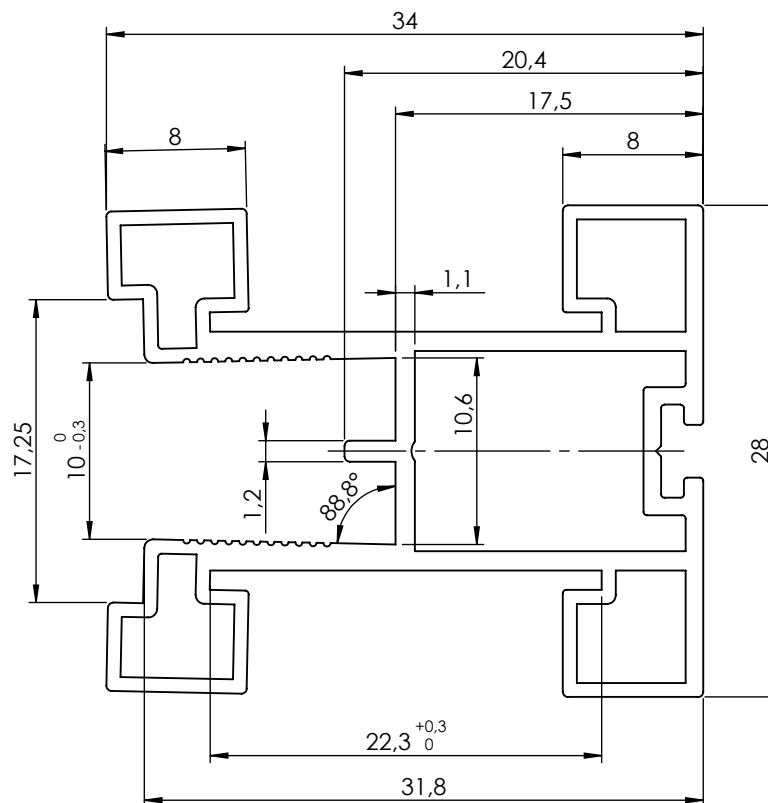
Aufrechtes Profil/Griffschiene BS Komfort Rahmentyp A/TOSCA 84000
